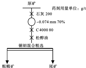
图 1 铜钼混浮条件试验流程
