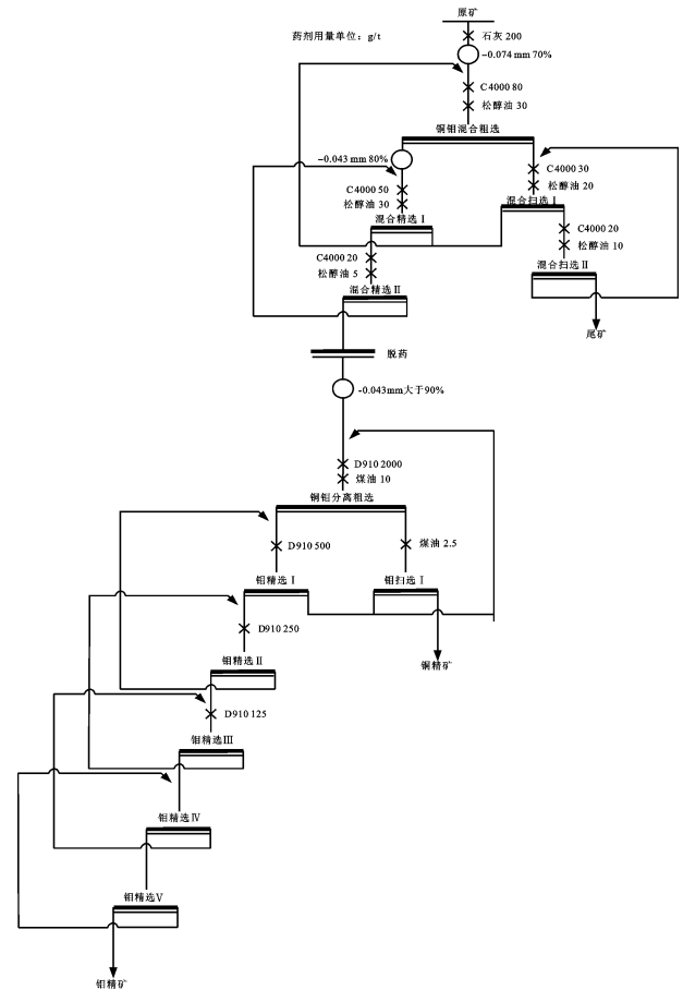
图3 闭路试验流程
