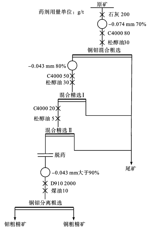
图 2 铜钼分离条件试验流程
