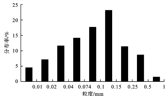
图1 金红石粒度统计
