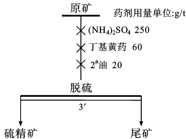
图1 浮选脱硫流程
