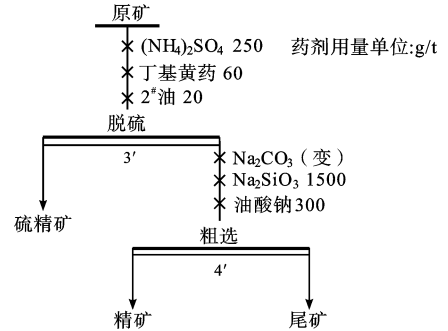
图2 碳酸钠用量试验流程
