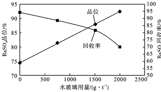
图 4 水玻璃用量试验结果
