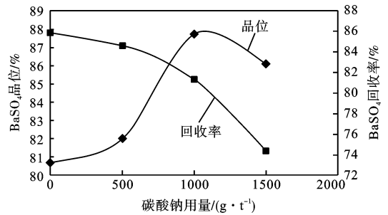
图3 碳酸钠用量试验结果
